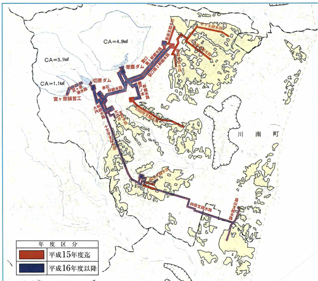
国営尾鈴土地改良事業計画一般平面図
